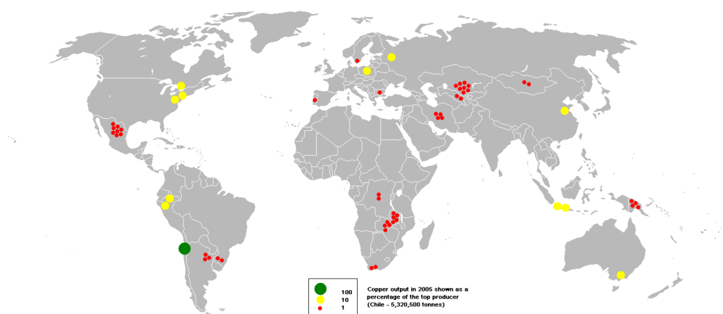
Figur 3.6 Kopparkopparproduktionen under 2005. Källa: http://en.wikipedia.org/wiki/Copper
